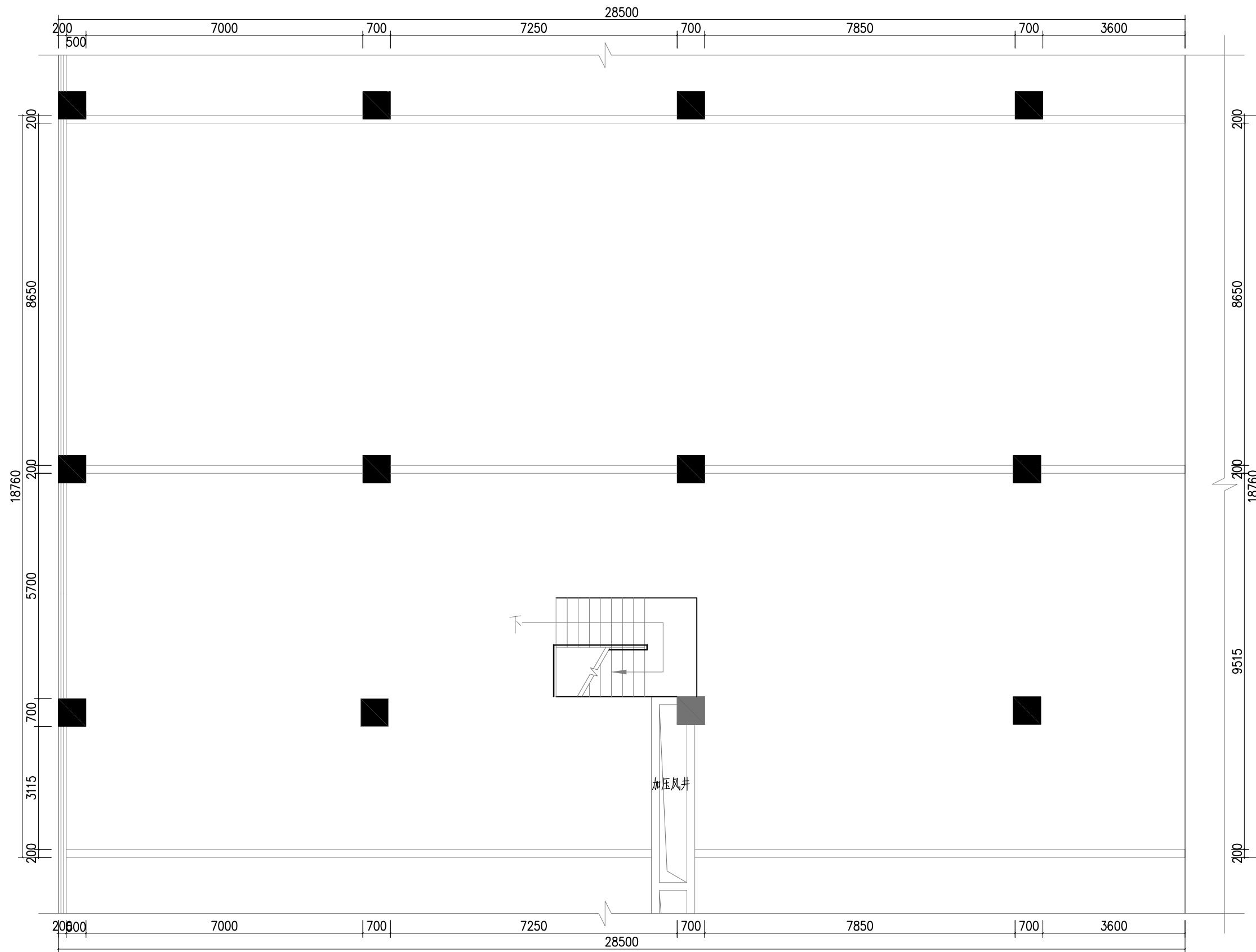
二层原始结构图 SCALE 1:75
