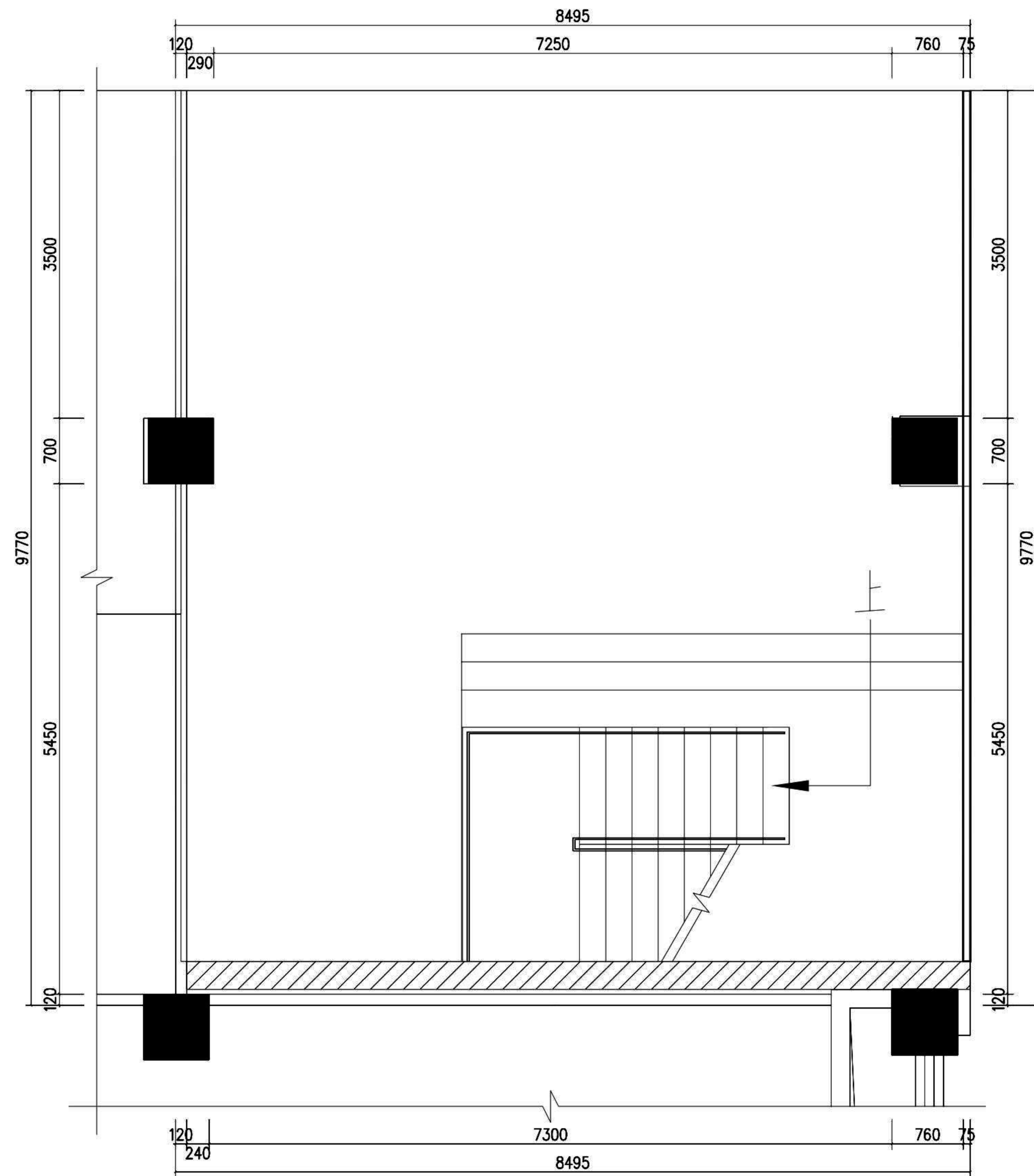
— 一层原始结构图 SCALE 1:40
